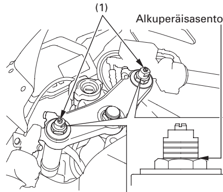
(1) Esijännityksen säätö
